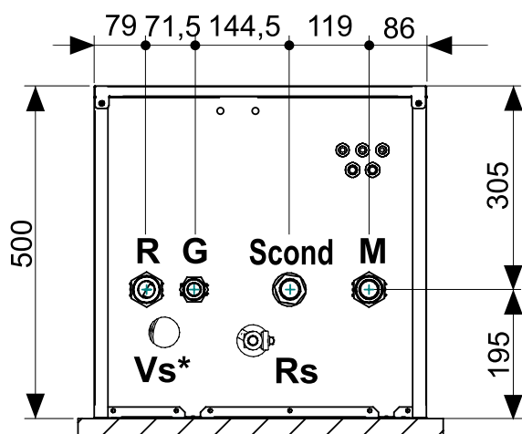
ВИД СНИЗУ
