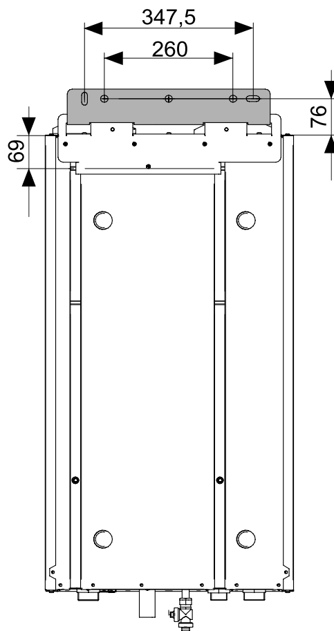
ВИД СЗАДИ
